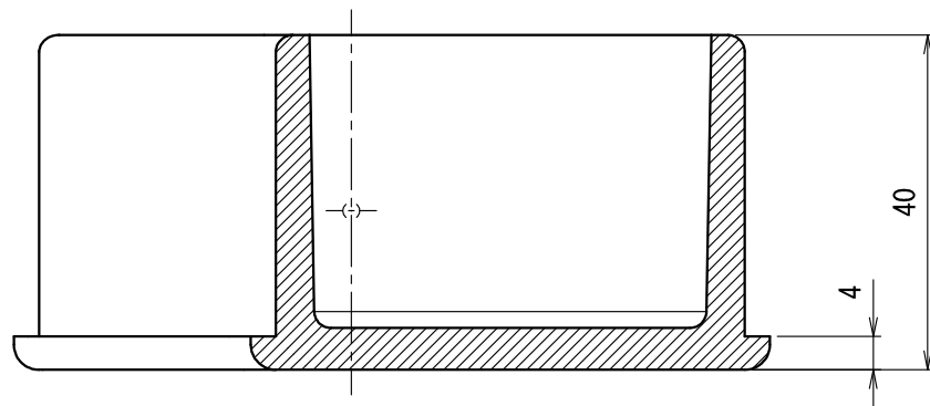
断面 A-A
